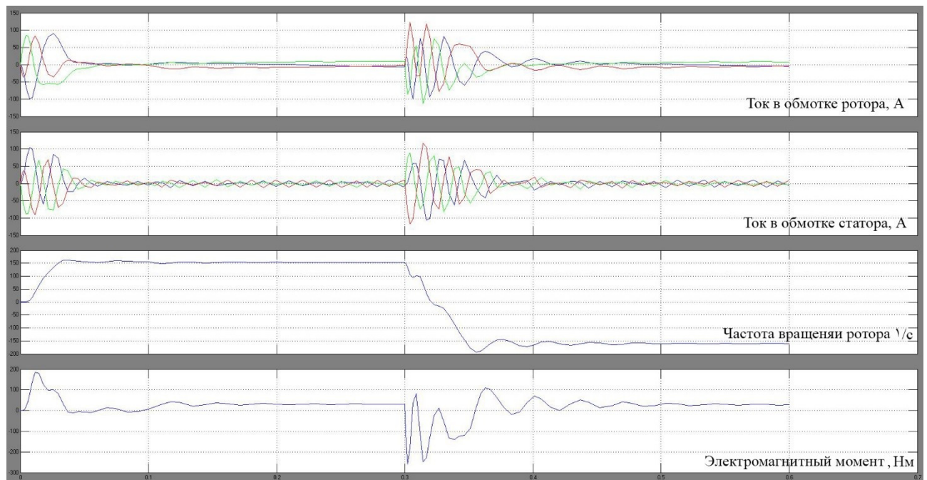
Рис. 3. Результаты моделирования пуска-реверса, зависимость токов от времени
