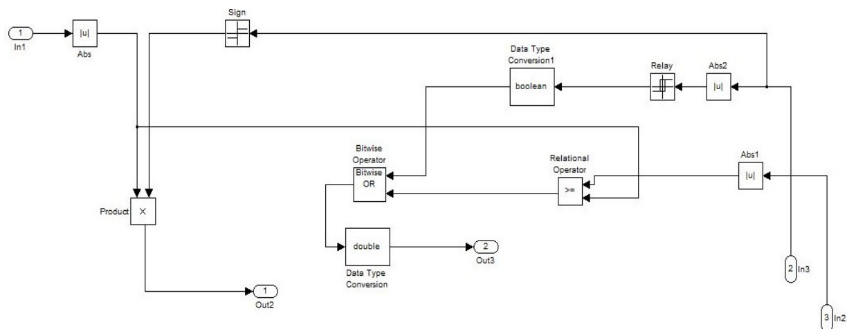
Рис. 7. Блок Subsystem
