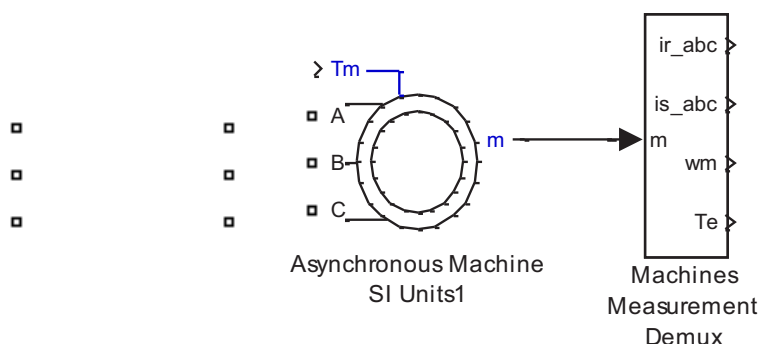
Рис. Ошибка! Текст указанного стиля в документе отсутствует.. Модель асинхронного двигателя библиотеки SimPowerSystems
