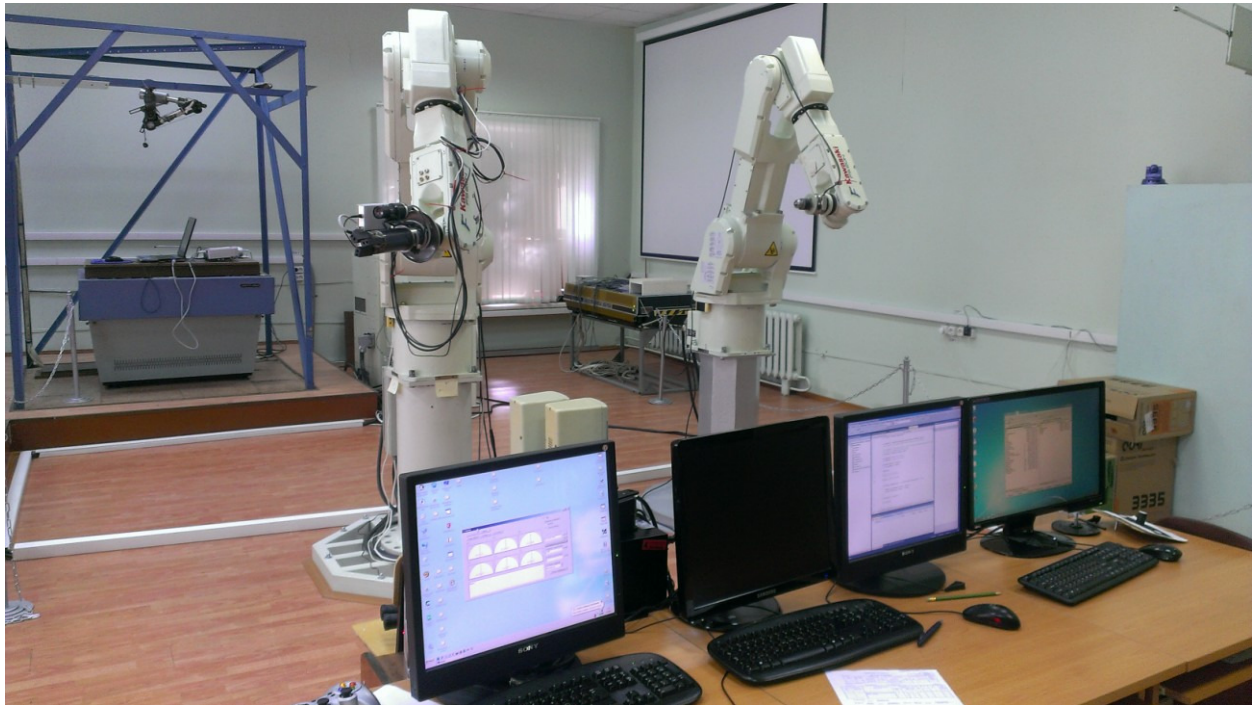
Рис. 2. Внешний вид станда для полунатурного моделирования КМР
